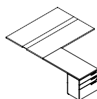
29 \frac{7}{8} " H (757 mm) C_N_-R____ELUF C_N_-R____ELF C_N_-R____UF
