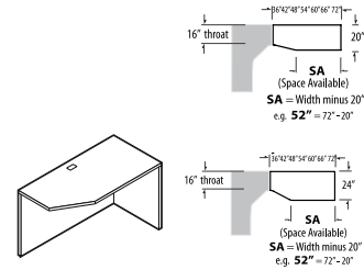
Space Saver Return - RIGHT*
